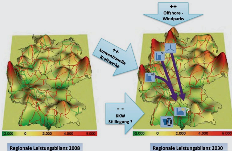
Abb. 3.11: „Regionale Leistungsbilanz“ – Die zunehmend verbraucherferne Konzentration von konventionellen Kraftwerken und zukünftig insbesondere Windparks, macht den Netzausbau erforderlich.
