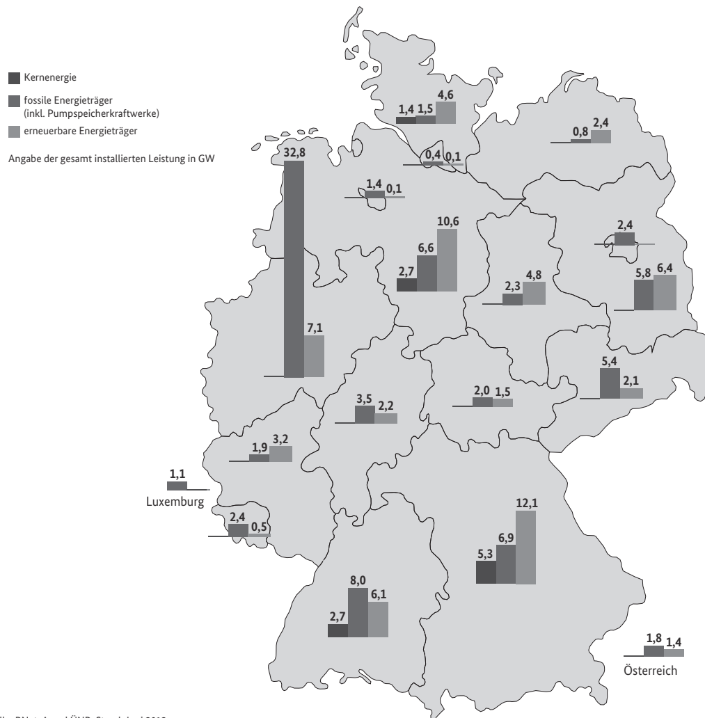
Abbildung 16: Die Verteilung der Kraftwerkskapazität auf die Länder
