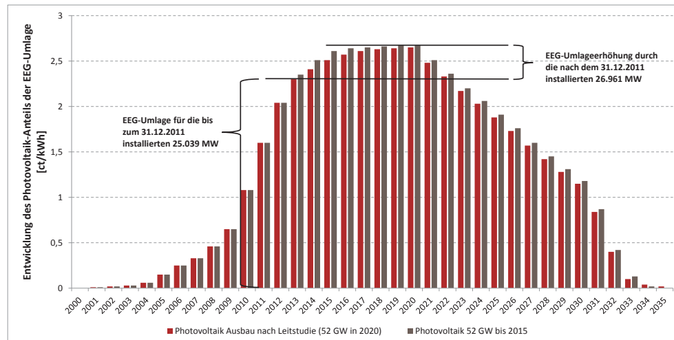
Abb. 4-5: Anteil der Photovoltaik an der EEG-Umlage bei Erreichen der 52 GW-Schwelle in 2015 bzw. 2020
