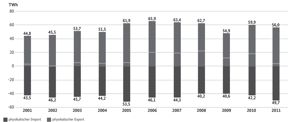
Abbildung 26: Die physikalischen Stromflüsse in den Grenzkapazitäten
