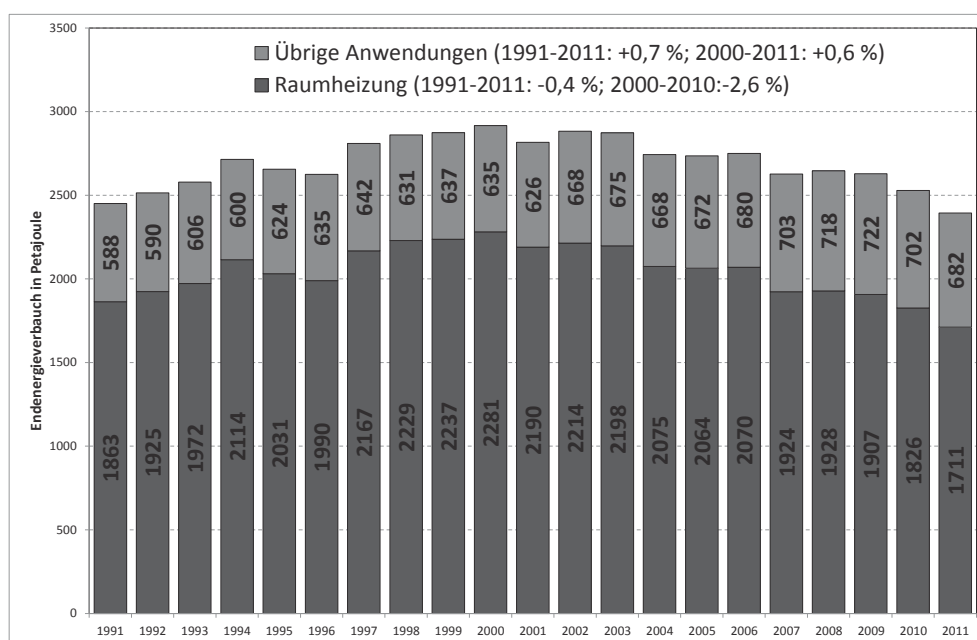
Abb. 3-7: Entwicklung des Endenergieverbrauchs der Haushalte nach Anwendungszwecken von 1991 bis 2011
