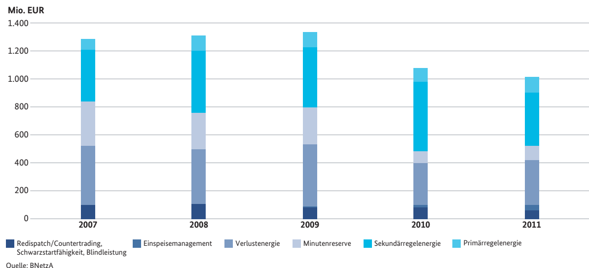
Abbildung 23: Kosten für Systemdienstleistungen
